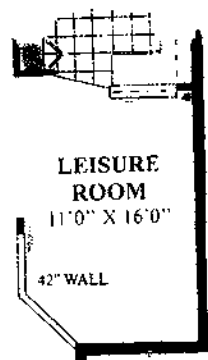
OPTION - A
